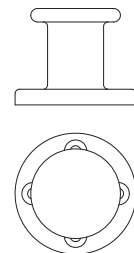
Тумбы Pillar
