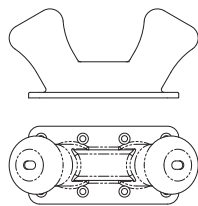
Тумбы Double bitt
